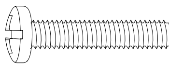
M-C (x4) M6x30
